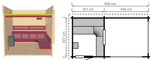
2 panneaux de verre coulissants, 1 porte sauna et 1 fenêtre sauna horizontale
