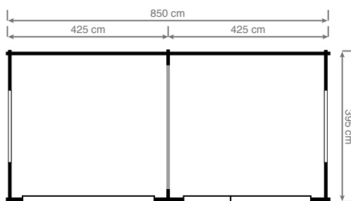
1 porte coulissante en aluminium, 1 grande fenêtre fixe en aluminium, 2 fenêtres fixes horizontales en aluminium
